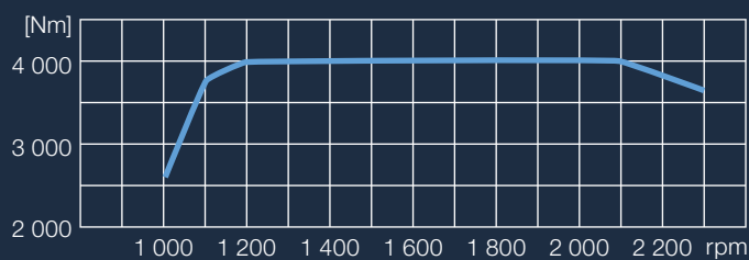
Torque V8-1200
